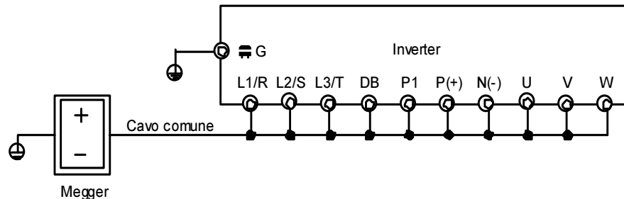
Figura 7-4-1 Test di isolamento
