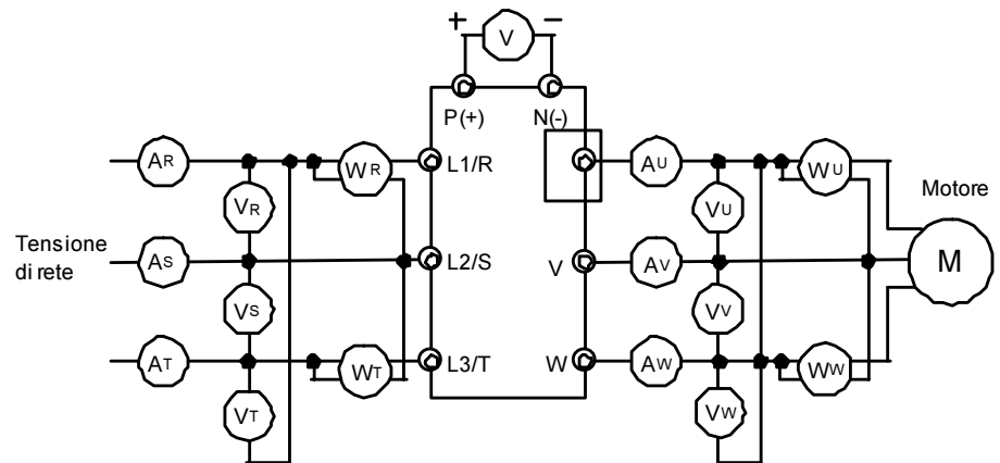
Figura 7-3-1 Cablaggio dei dispositivi di misurazione
